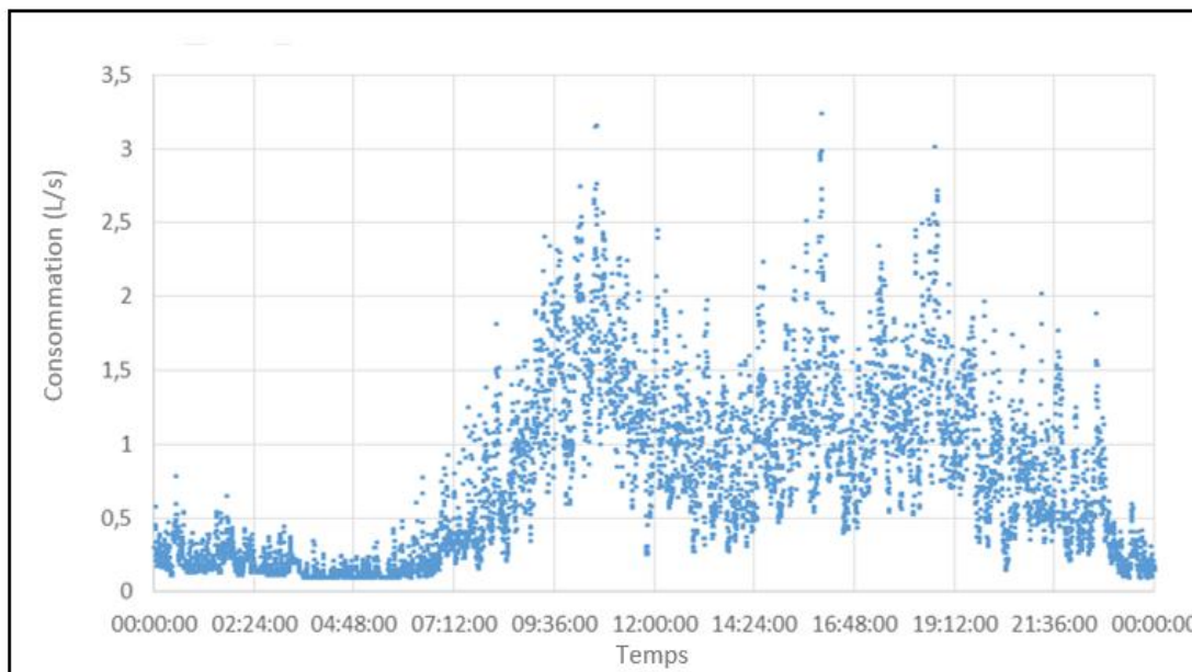
Figure 7. Débit entrant d'un SSC de 115 résidences unifamiliales à Saint-Georges (5 février 2017)
