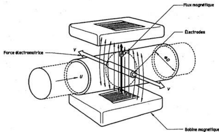
Figure 32. Principe de Faraday
