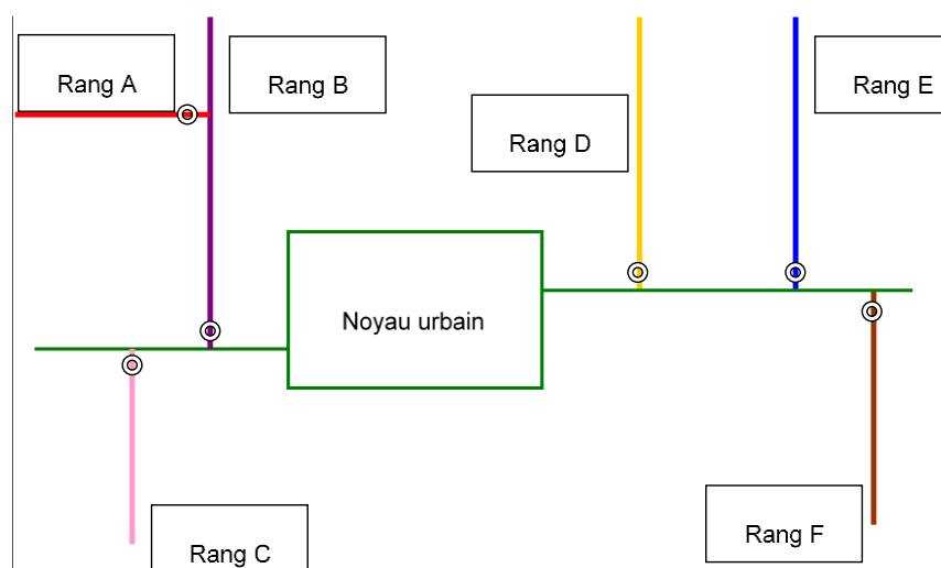
Figure 34. Exemple d'un réseau avec ses points de mesure
