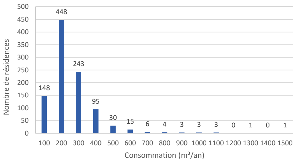
Figure 4. Histogramme de 1 000 consommations de résidences unifamiliales (Charlemagne)
