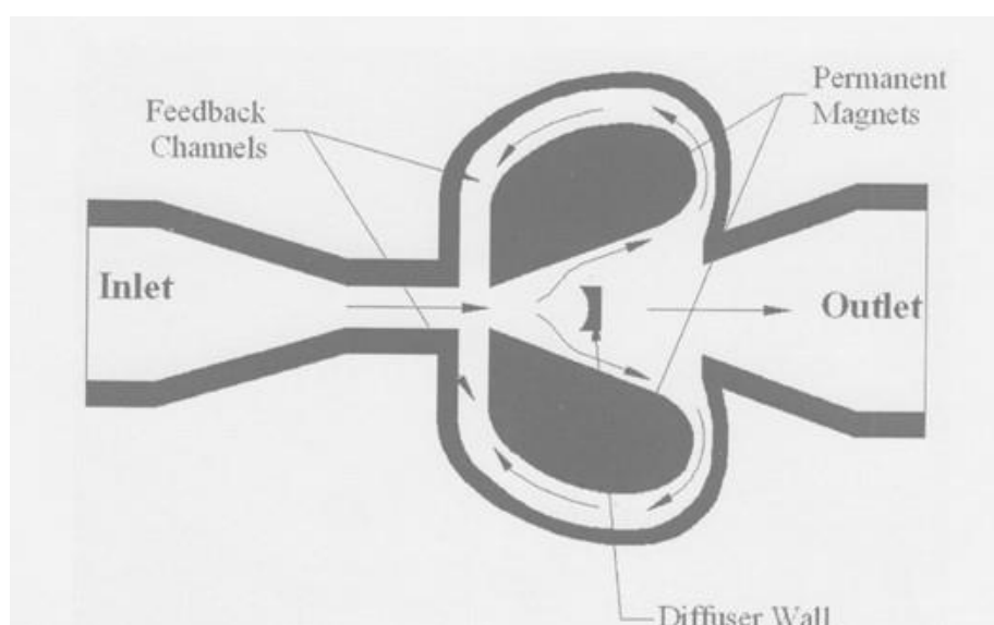
Figure 31. Compteur à oscillation fluide
